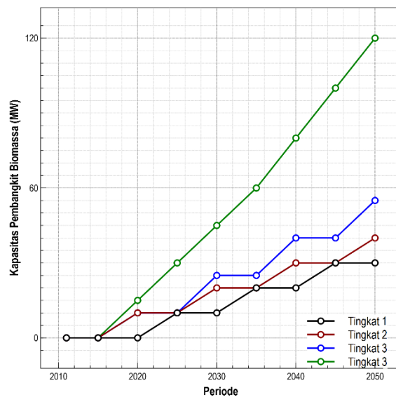
Gambar 1: Proyeksi kapasitas PLT biomassa
